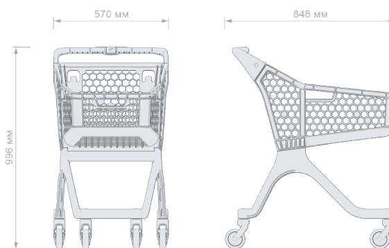
Габариты изделия
